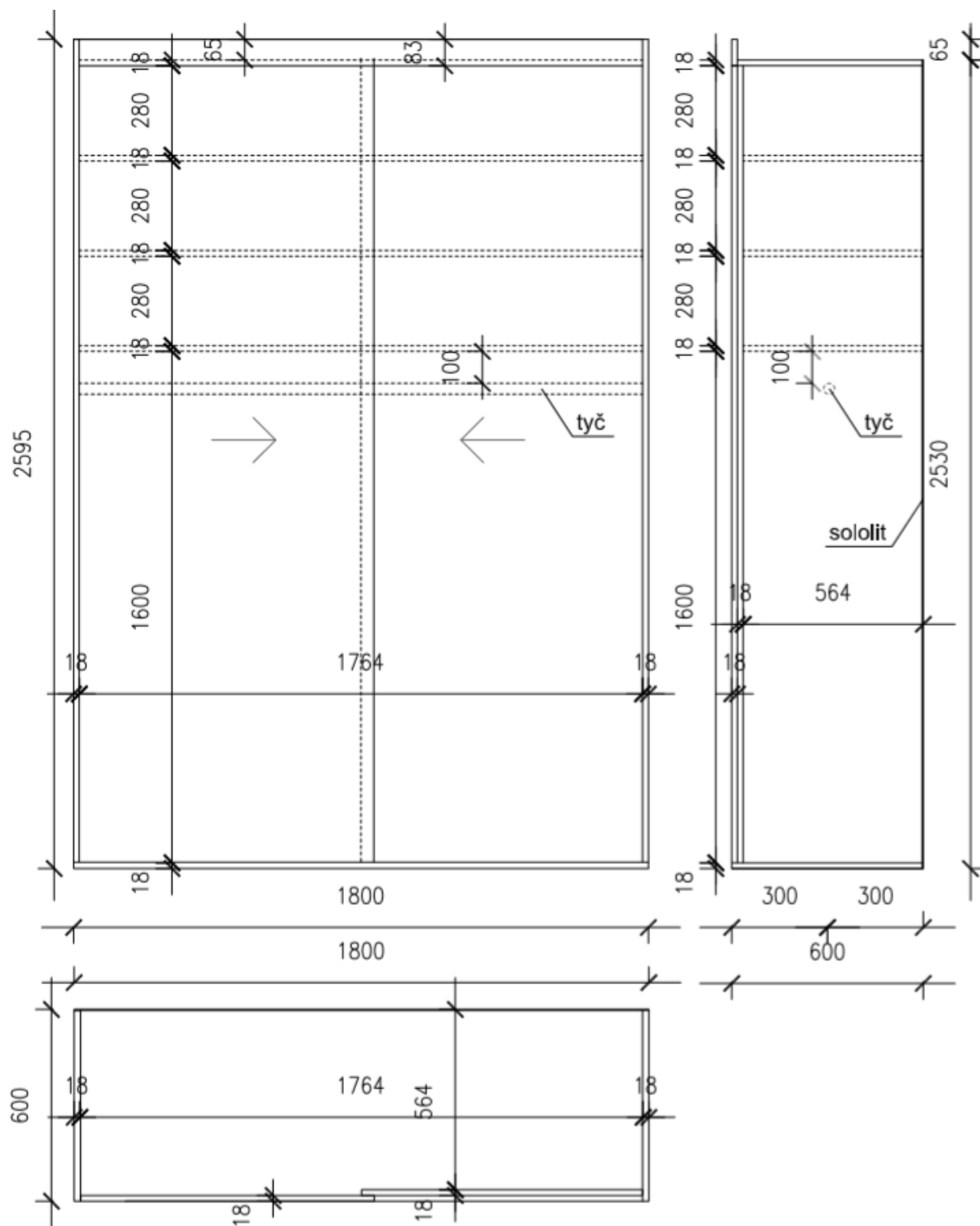
Šatní skříň
